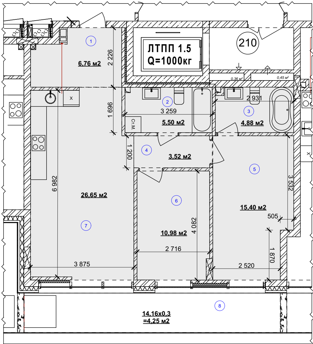
План 2 кімнатної квартири №42
