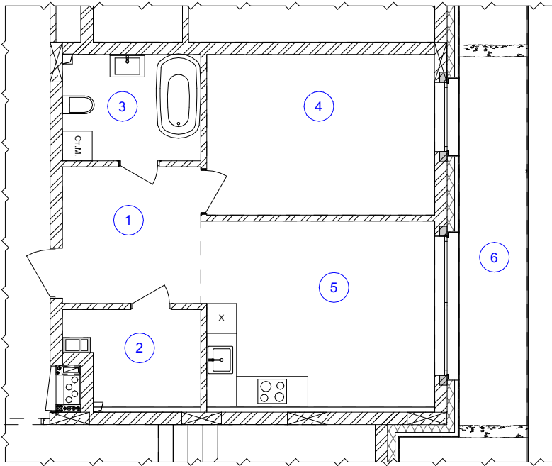
План 1- кімнатної квартири № 109
