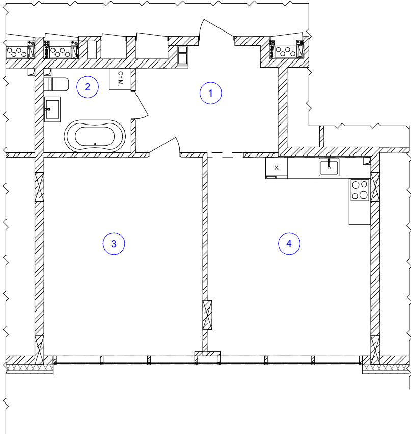
План 1- кімнатної квартири № 112
