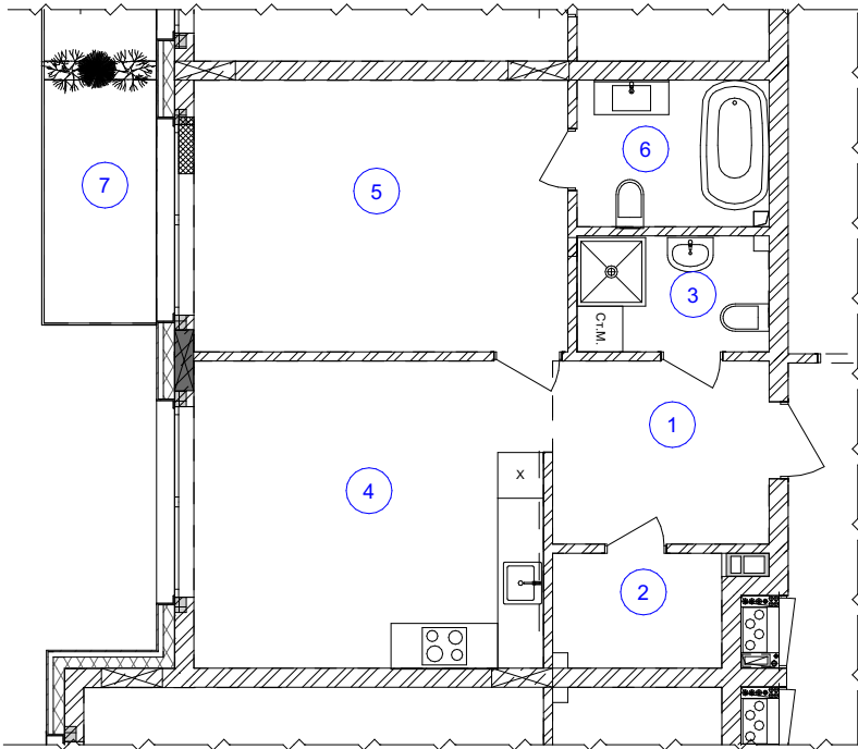
План 1- кімнатної квартири № 115
