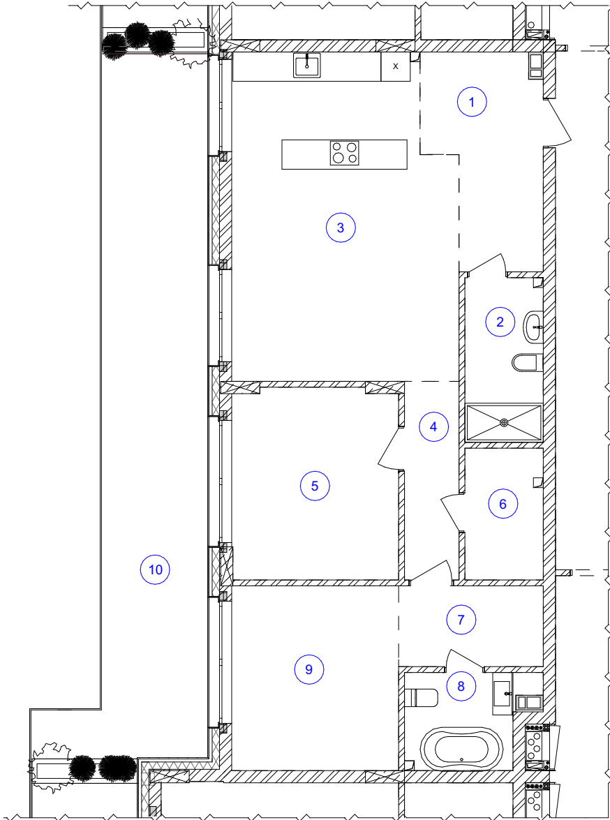
План 2- кімнатної квартири № 126
